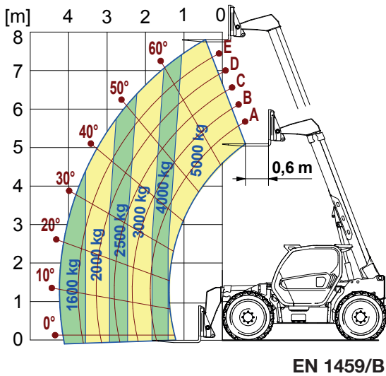
TF50.8 MET VORKEN TF50.8 AVEC FOURCHES
