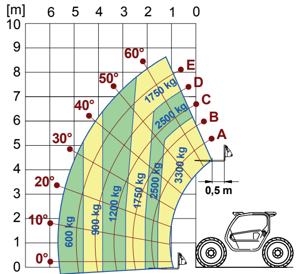
TF33.9 MET VORKEN EN 1459/B TF33.9 AVEC FOURCHES
