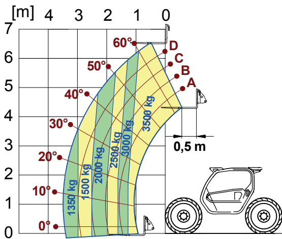
TF35.7 MET VORKEN EN 1459/B TF35.7 AVEC FOURCHES
